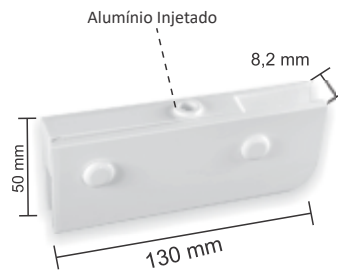
Dobradiça pivotante superior para 1009
