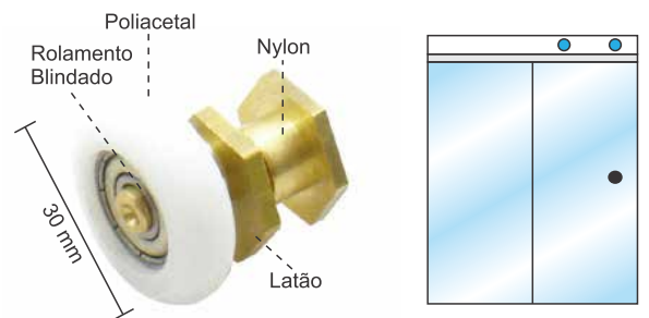
Roldana excêntrica para Box
