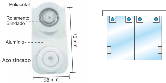
Mini carrinho simples para 1030 (1 furo, porta até 20kg)
