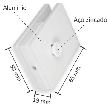
Grapa para sacada 50x65mm (Sem recorte)
