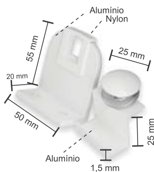
Conjunto acessório V/A para haste 1587
