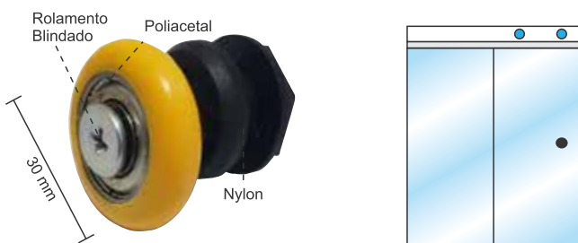
Roldana excêntrica corpo em nylon para Box
