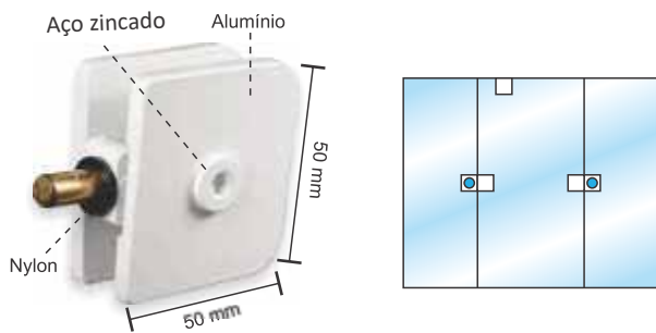
Dobradiça para basculante 50x50mm
