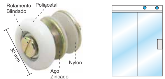
Roldana para porta e janela de correr
