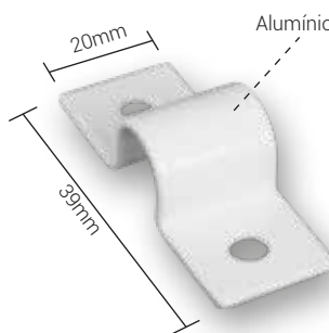
Contra trinco para 1519 e 1521
