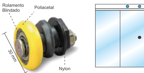
Roldana excêntrica para porta e janela de correr
