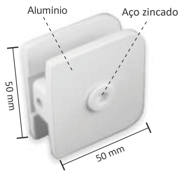
Suporte central para fixação 50x50mm
