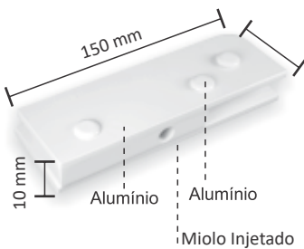
Dobradiça pivotante inferior para 1014
