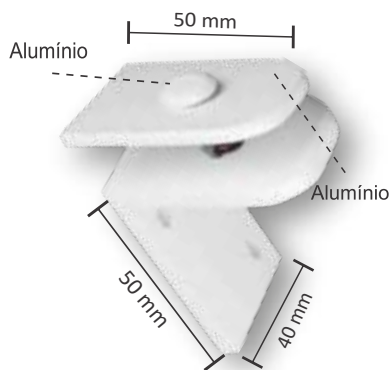
Suporte para prateleiras
