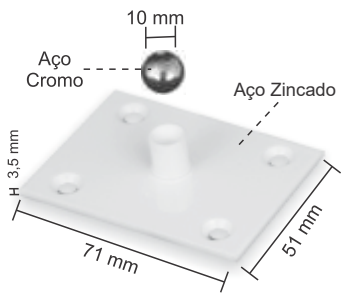
Max pivô inferior para dobradiça 1102G
