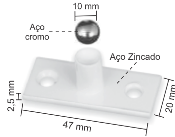
Pivô inferior para dobradiça 1102
