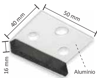
Batedeira para trinco de basculante
