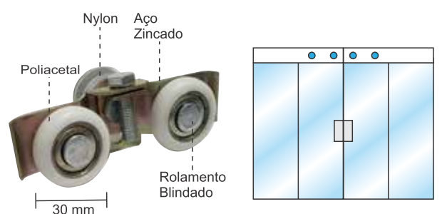
Roldana dupla com regulagem
