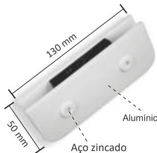
Suporte de centro com rosca para roldana 1150
