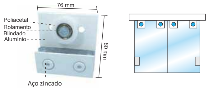
Carrinho simples para 1030 (2 furos, porta até 30kg)
