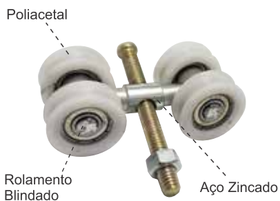
Roldana quadrupla para trilho 1030
