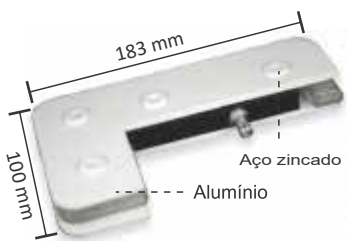
Facão simples para bandeira e fixo para 1101
