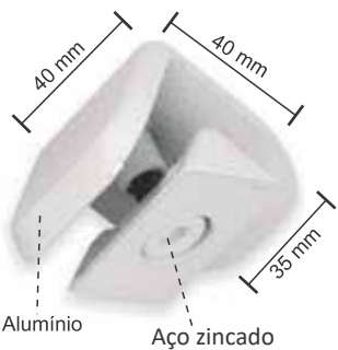
Suporte de centro com núcleo para união de 2 vidros à 90°
